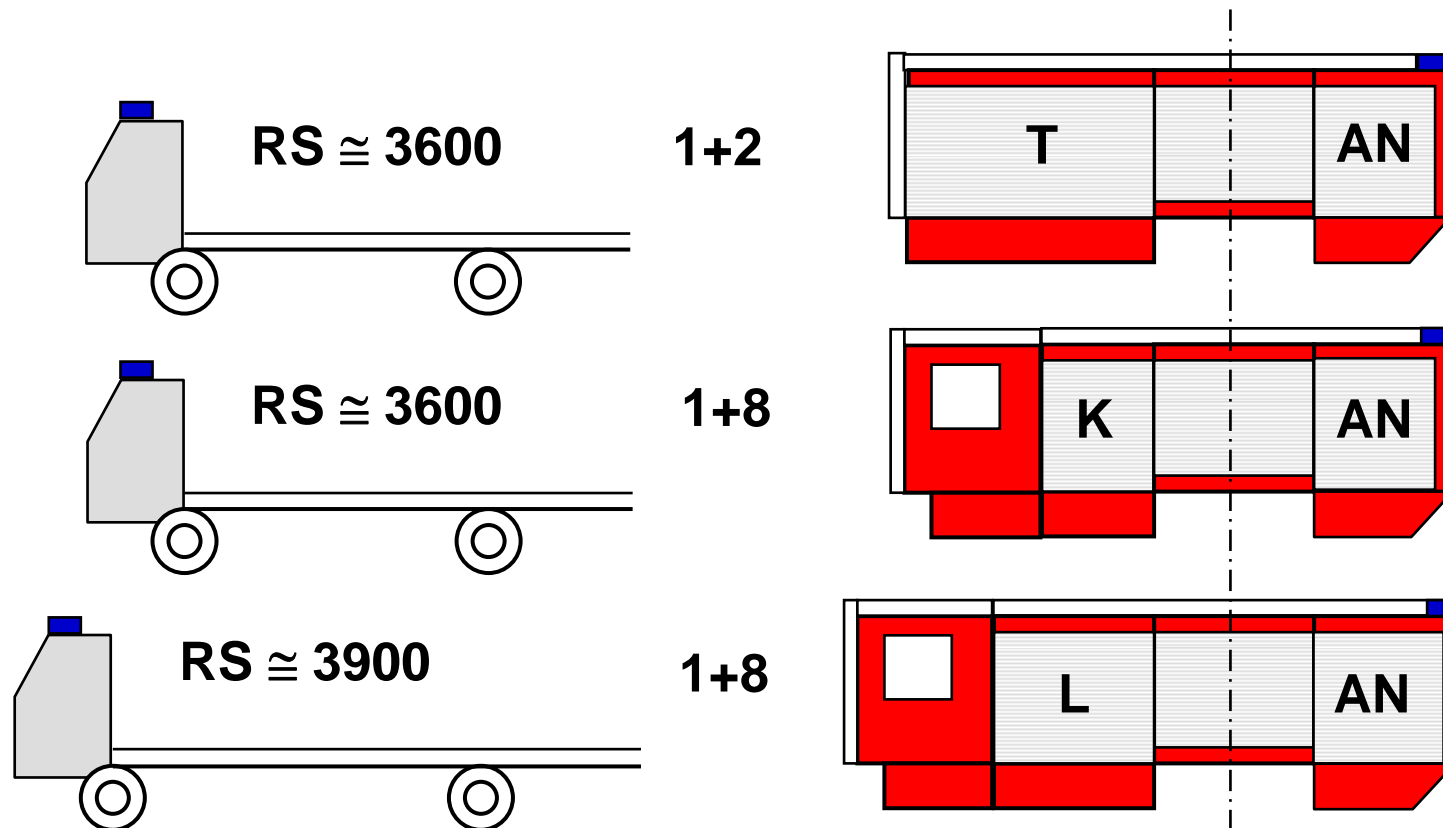
Aufbauvarianten AT
